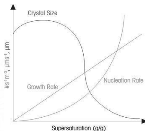
Gambar 2.1 Hubungan antara supersaturasi dengan laju nukleasi, pertumbuhan kristal dan ukuran kristal (O'Sullivan dkk, 2012)
